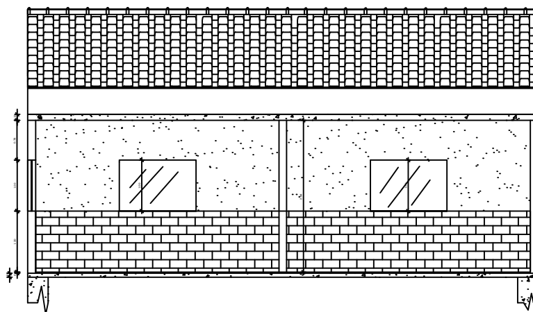
ARQ-SALA-CORTE -A ESC: 1/100
