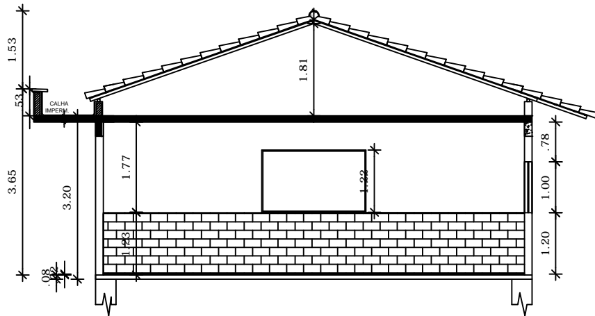
ARQ-SALA-CORTE - B ESC: 1/100
