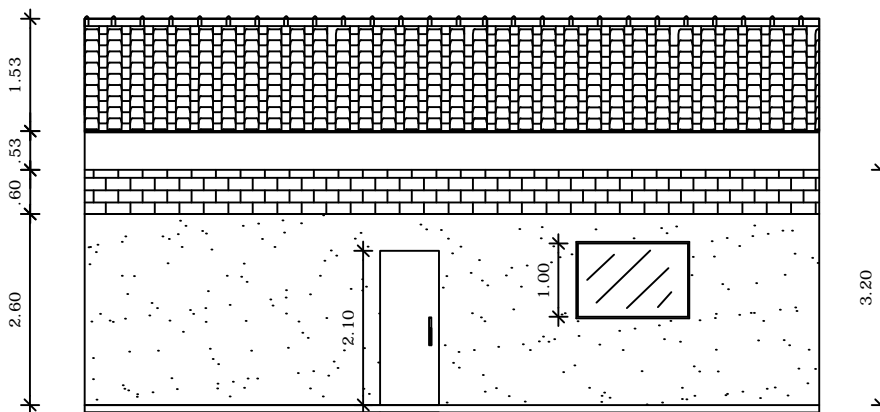
ARQ-SALA-VISTA1 ESC: 1/100
