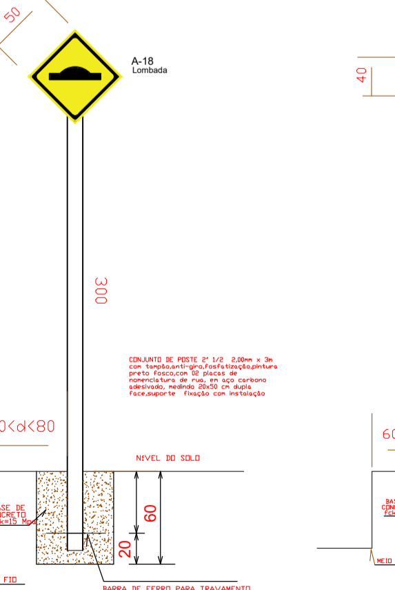
DETALHE PLACA A-18 - SEM ESCALA
