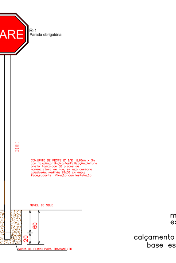
DETALHE PLACA R-1 - SEM ESCALA
