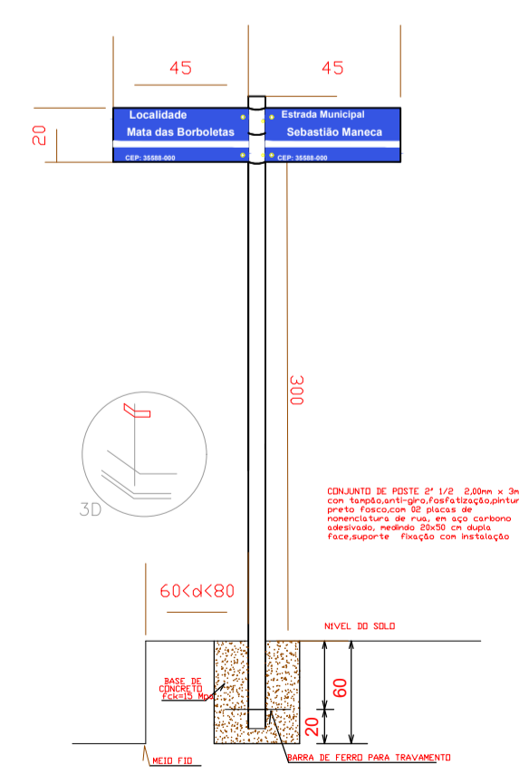
DETALHE PLACA ID - SEM ESCALA
