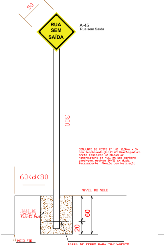
DETALHE PLACA A-45 - SEM ESCALA
