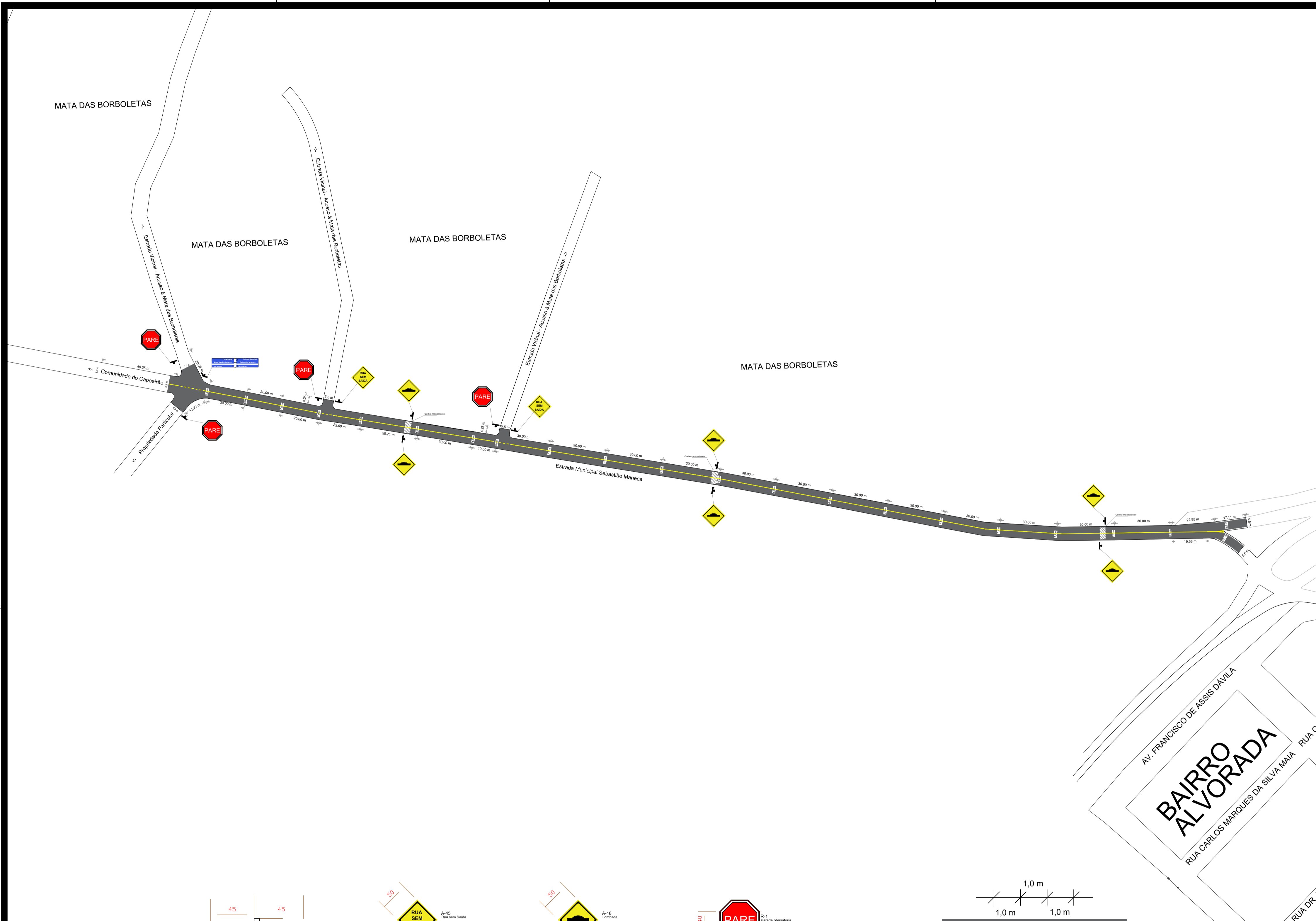
DETALHE SIN. HORIZONTAL - SEM ESCALA
