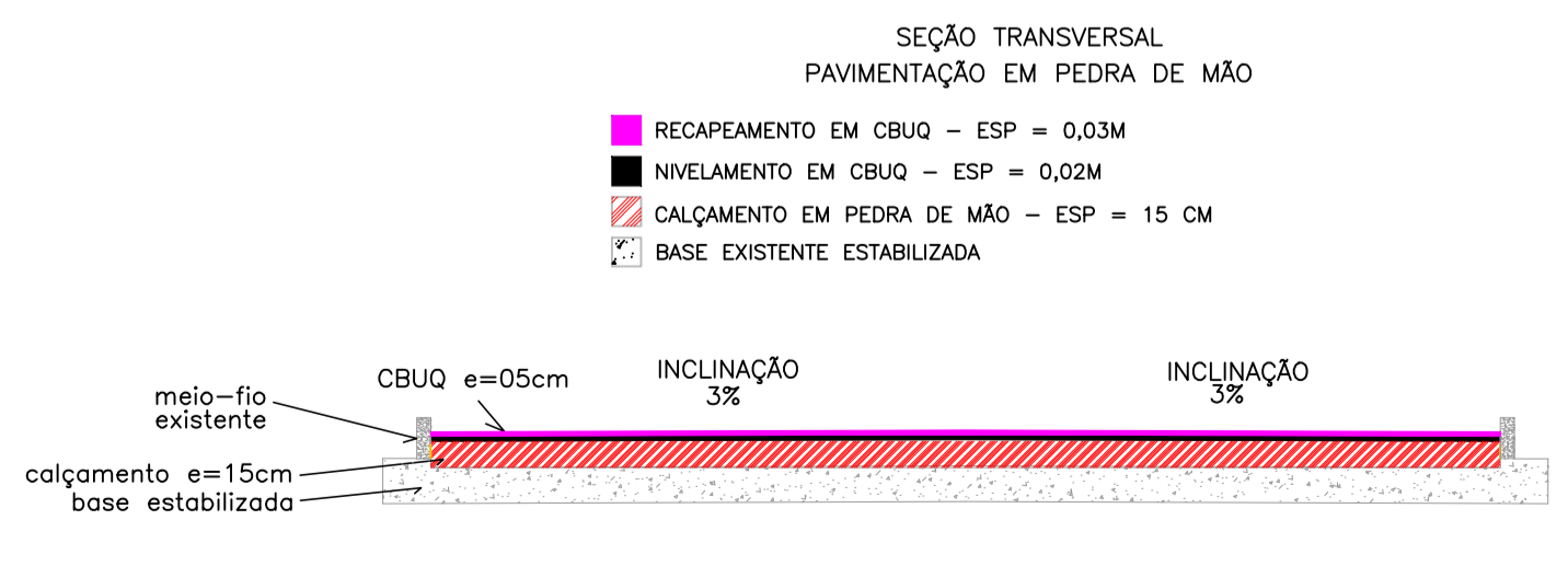
DETALHE SEÇÃO DA VIA - SEM ESCALA
